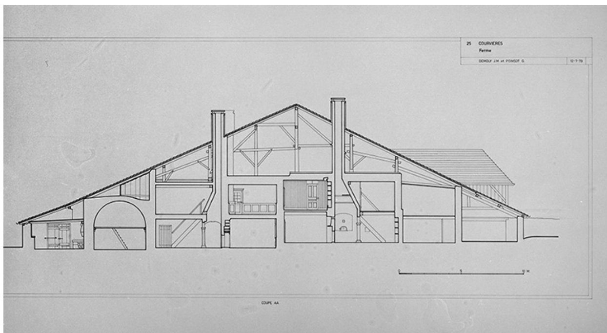
Coupe transversale d'une ferme.
