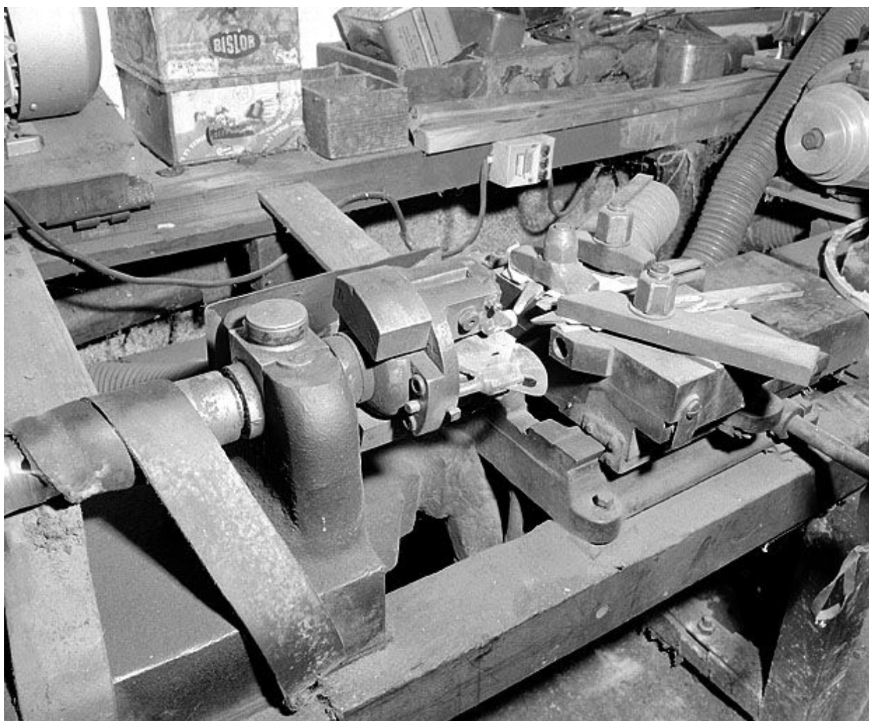
Mandrin gueule de loup et chariot porte-outils.
