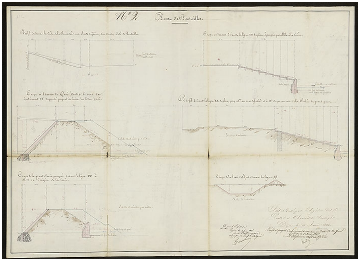
Port de Pontailler. [Coupes et profils]. 1835.
