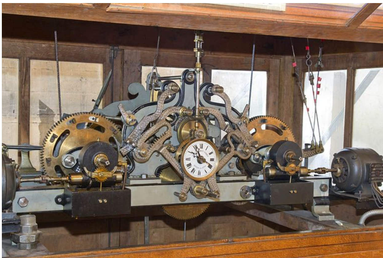
Mécanisme de l'horloge d'édifice L.-D. Odobey Cadet donnée en 1933 par Albert Odobey à l'Ecole nationale d'Optique.
