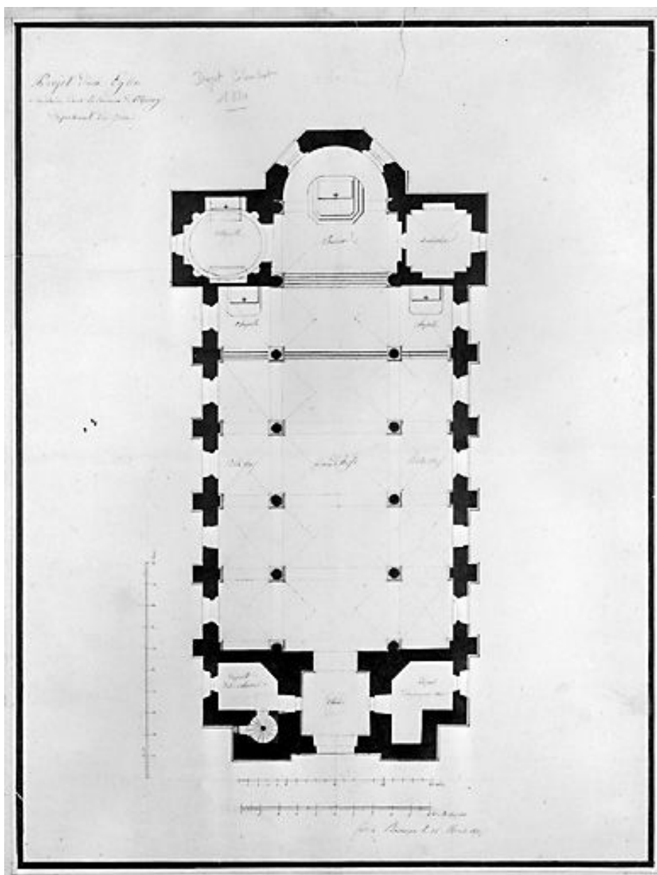
Projet d'une église à construire dans la commune de Morey, 1810. Dessin (plume, lavis), 14 mars 1810.
