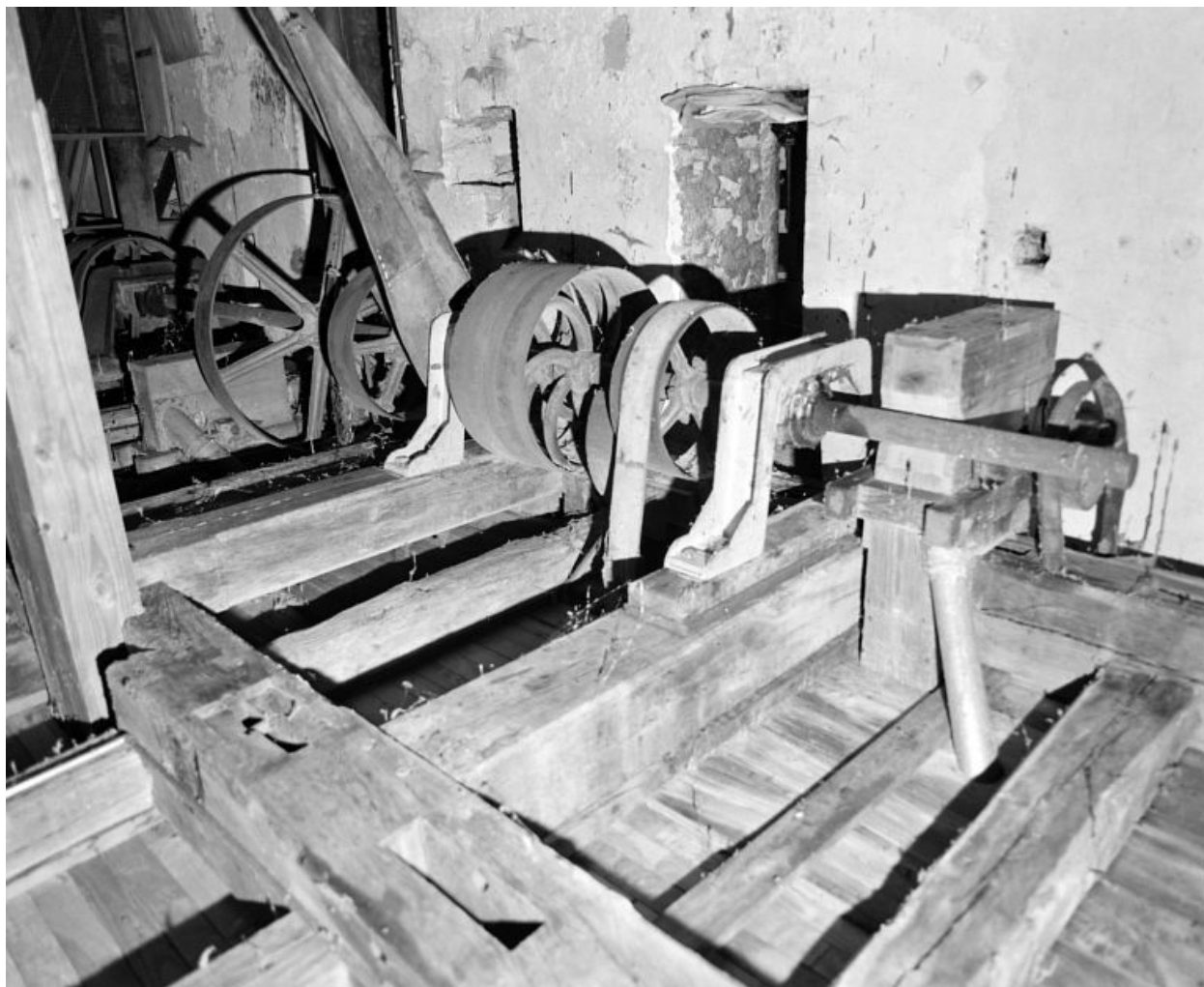
Rez-de-chaussée. Arbre de transmission et poulies.
