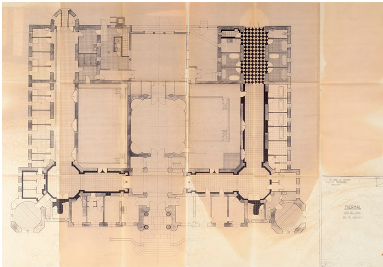
Plan du rez-de-chaussée avant les travaux (14 septembre 1981).
