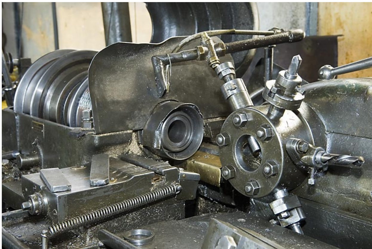
Tour à décolleter Loewe & Co (N). Détail du barillet porte-outils.
