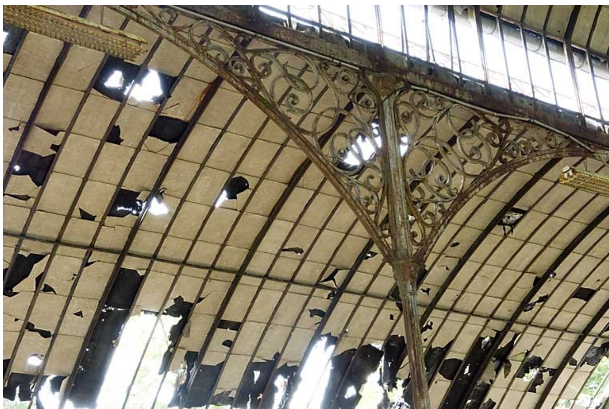
Intérieur de la serre. Console de la charpente métallique.
