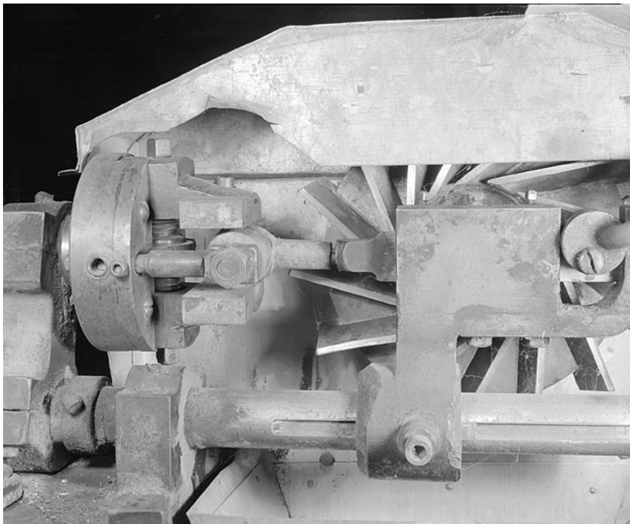
Le mandrin "gueule de loup".
