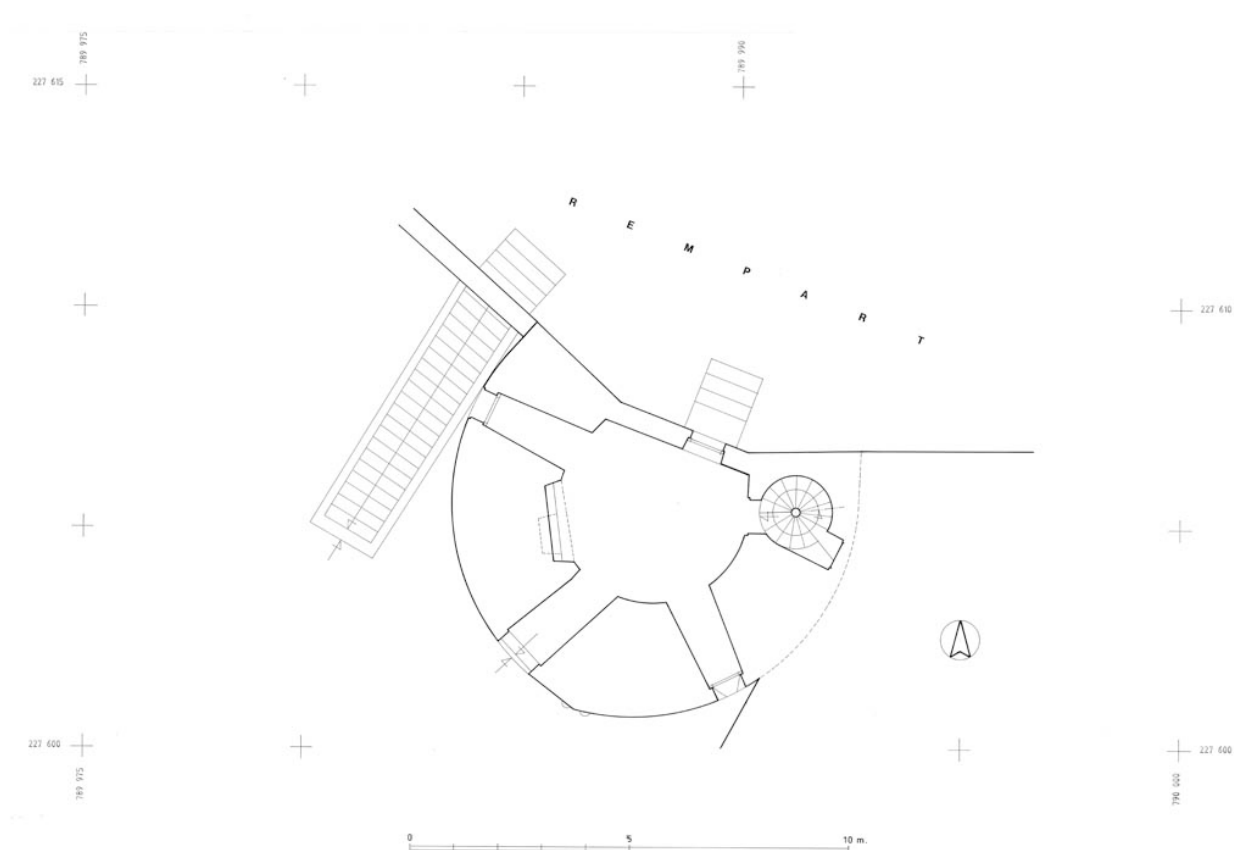
Tour des Cordeliers. Plan du troisième niveau.
