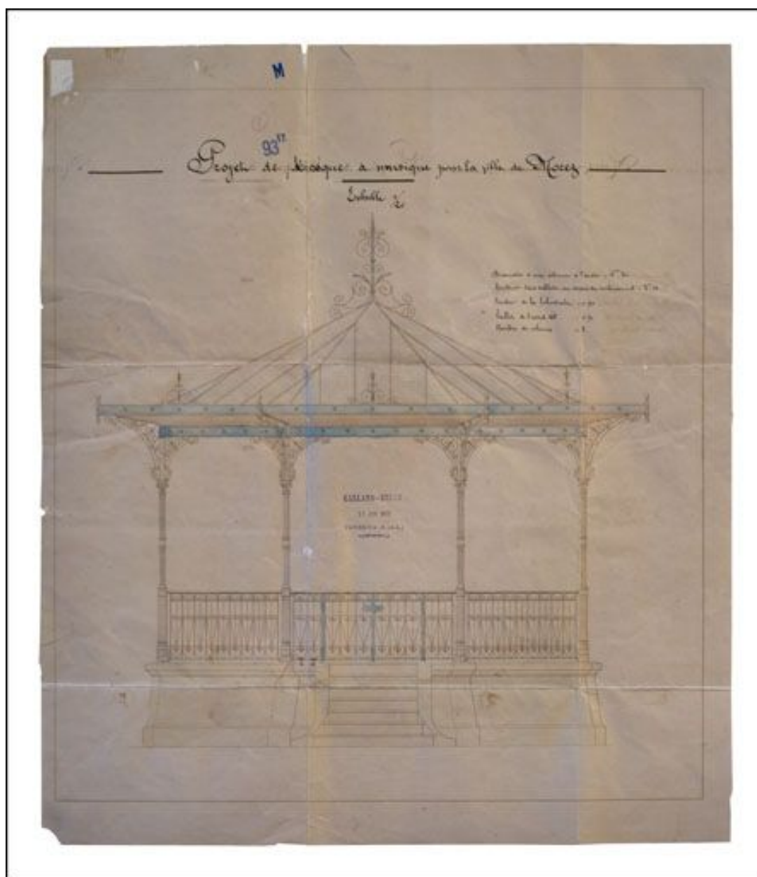
Projet de kiosque à musique pour la ville de Morez : dessin (tirage à l'ammoniaque rehaussé de lavis), 15 juin 1899, échelle 1:20.
