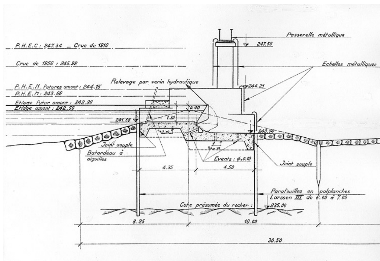
Barrage de la Malate. Equipement avec bouchure mobile. Coupe transversale du barrage (partie mobile), 1959.
