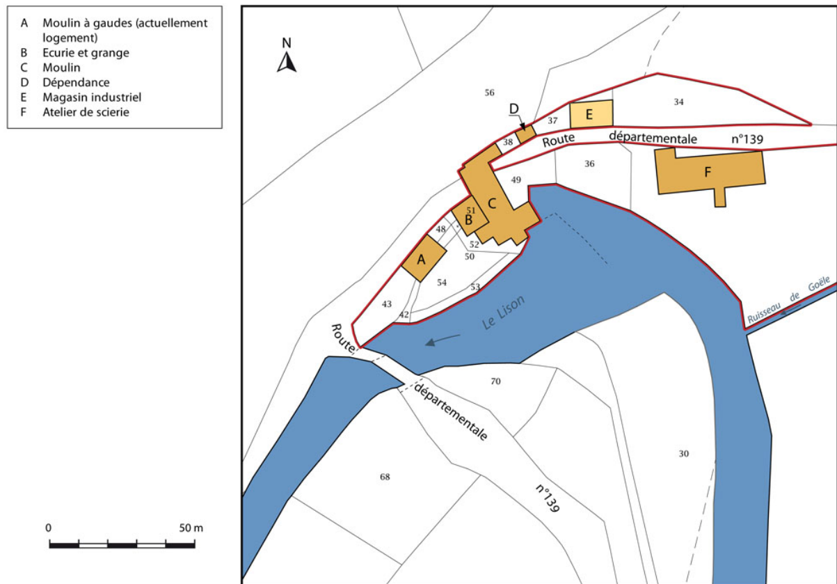
Plan-masse et de situation. Extrait du plan cadastral, 2015, section ZD.
