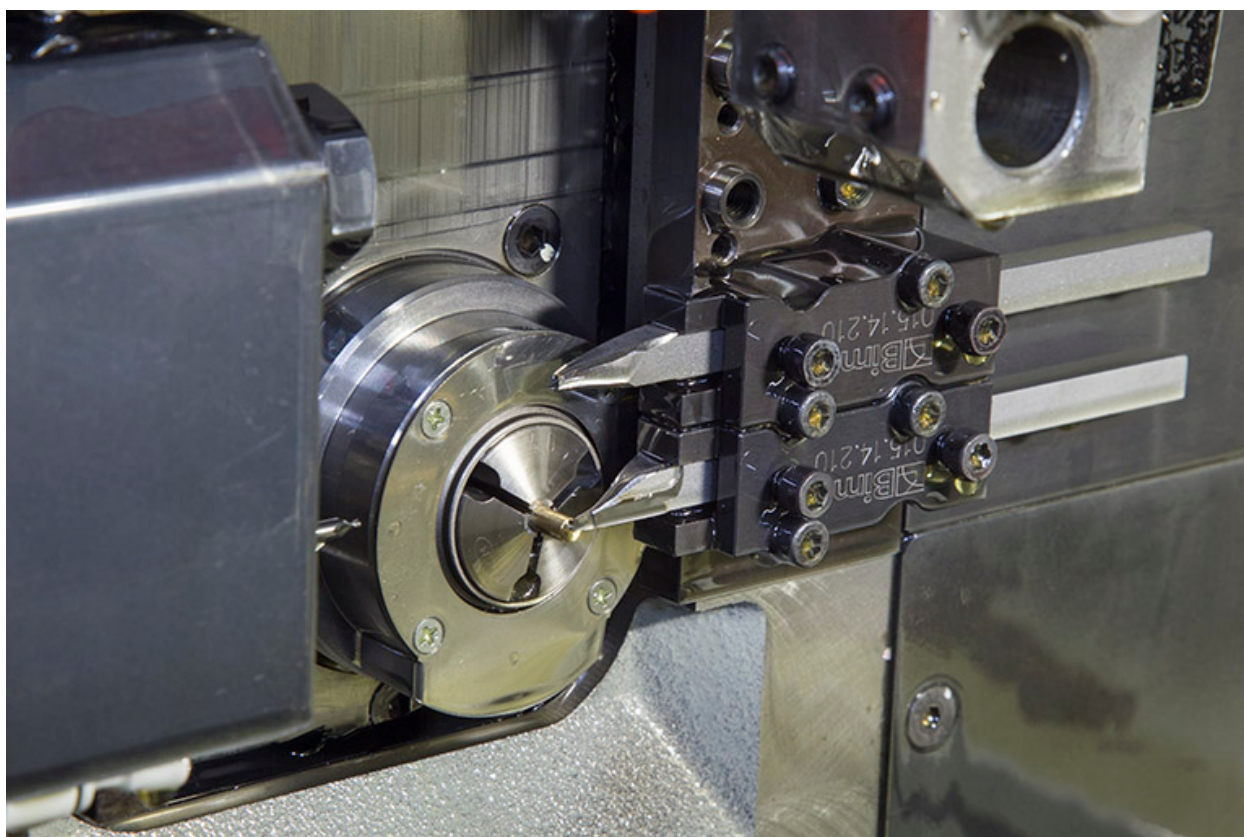
Machine à décolleter récente : pièce et outils.
