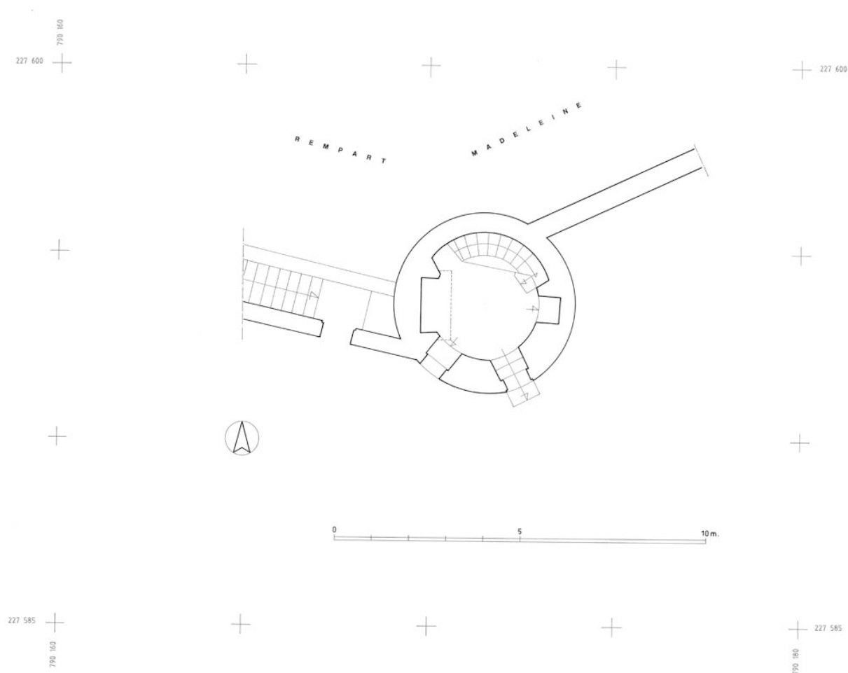
Tour des Billes. Plan du niveau supérieur.
