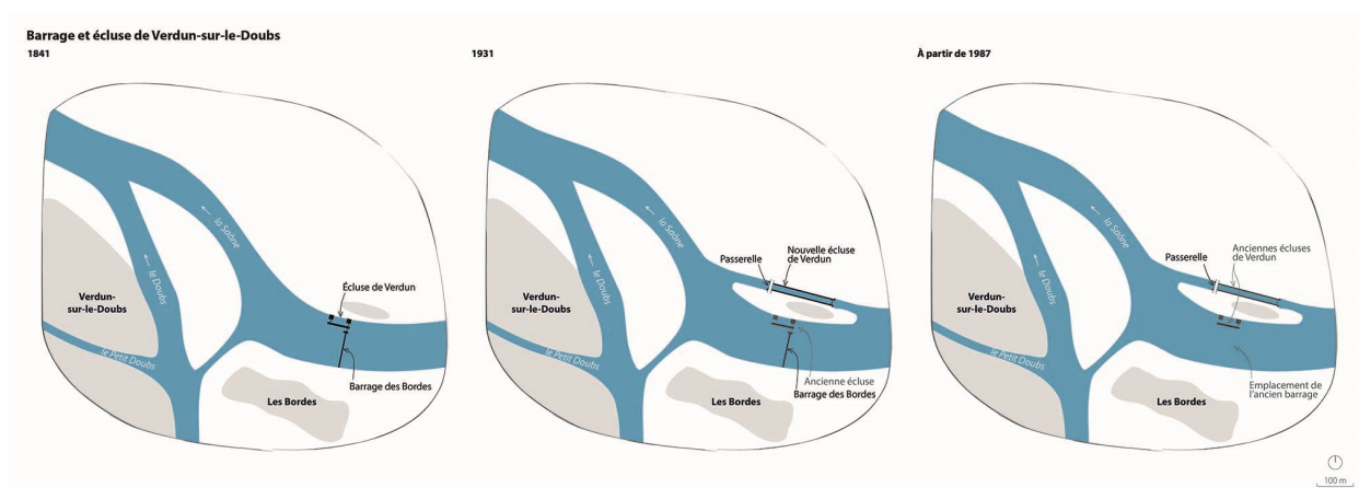
Plans schématiques (en 1841, 1931 et dès 1987) du barrage et de l'écluse de Verdun-sur-le-Doubs, échelle 1 / 5 000e.
