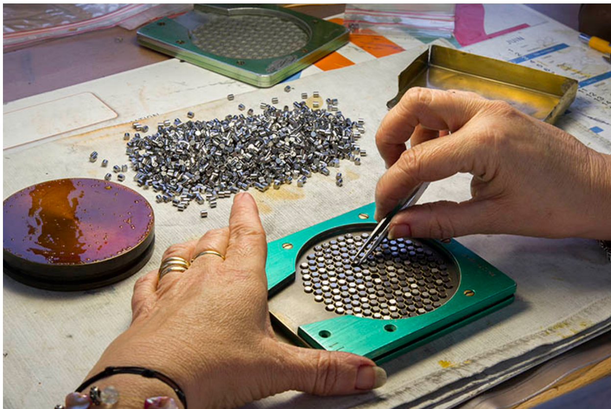
Atelier de polissage : mise en place des pièces sur un plot.
