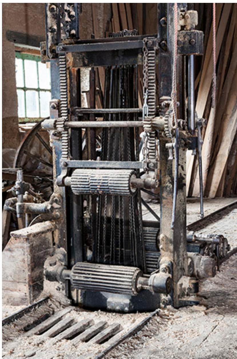
Scierie des Mortes, Chapelle-des-Bois (les Mortes) : châssis de scie multilame Benier-Rollet.
