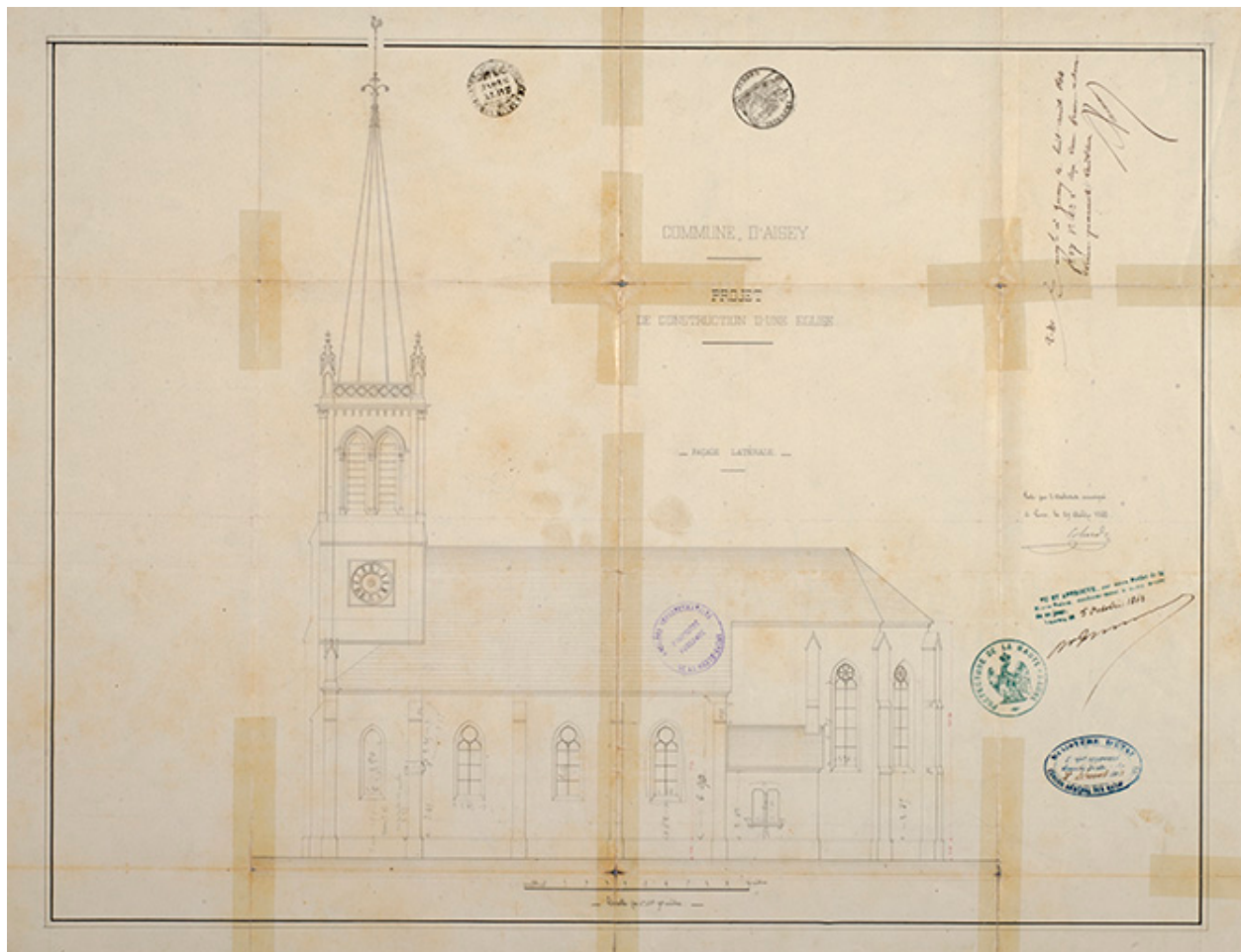
Projet de construction de l'église, façade latérale (1862).
