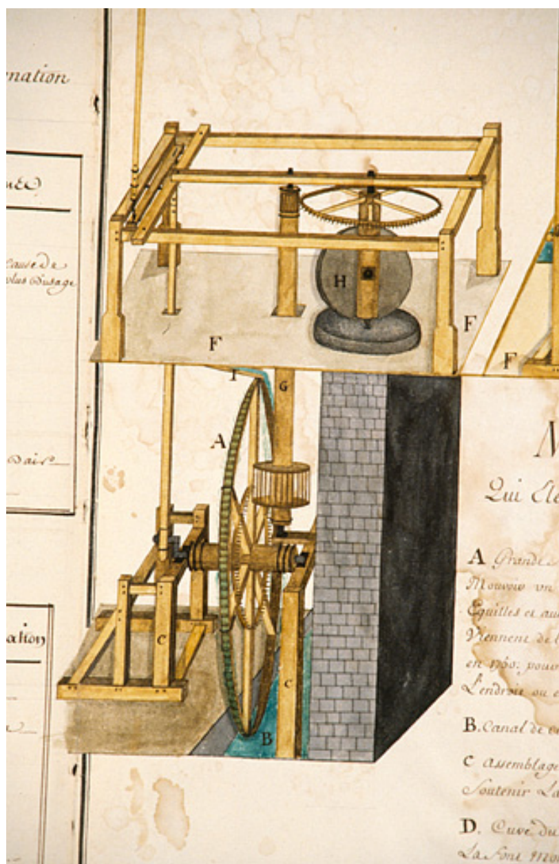
Machines Hydrauliques Qui Elèvent les Eaux de la cuve du Tripot [détail de la roue hydraulique et de la meule verticale], dessin, 1756.
