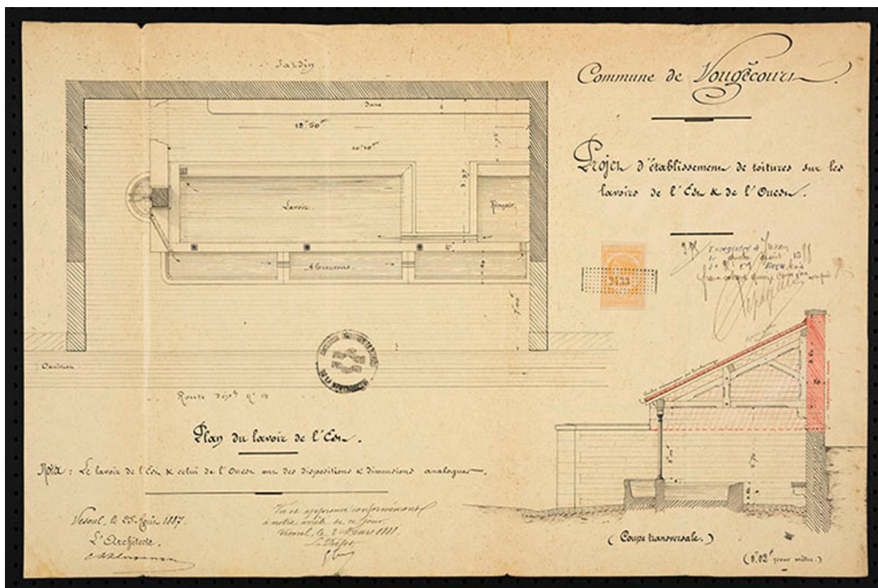
Projet d'établissement de toitures sur les lavoirs. [plans et coupes] 1887
