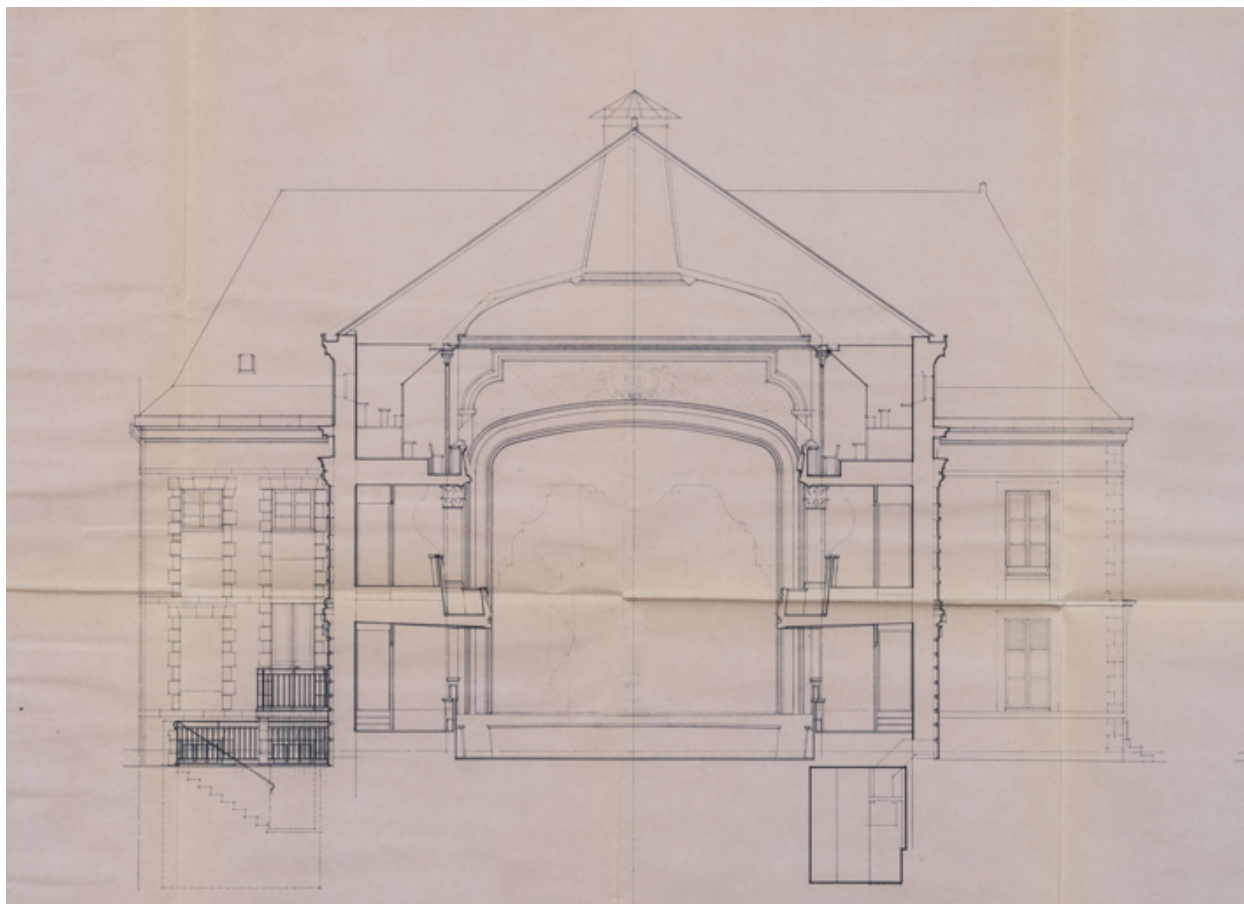
Théâtre municipal. Mise en conformité. Rénovation. APD. SC 8A. Coupes transversales sur salle et sur scène [détail : coupe sur la salle]. 1978.
