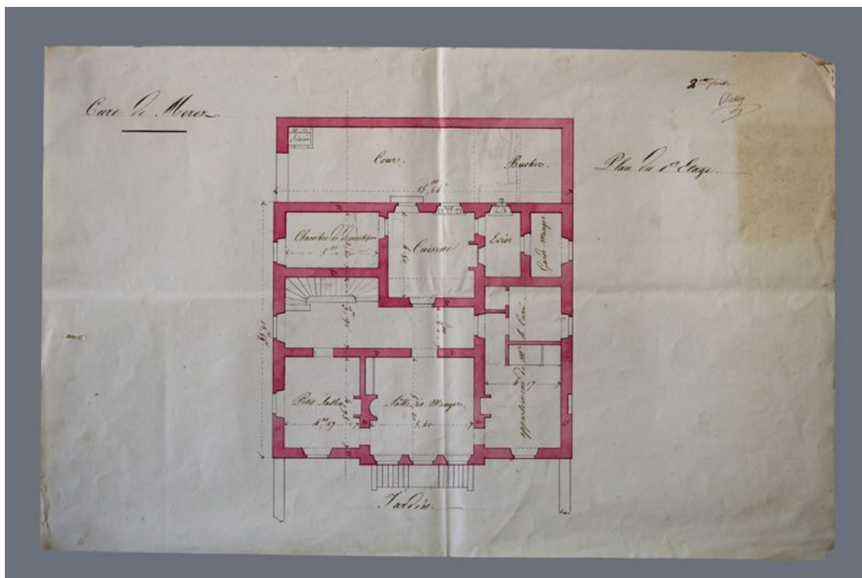
Cure de Morez. 2e feuille. Plan du 1er étage, 1836. Dessin (plume, lavis), [mars] 1836, sans échelle [1:100].
