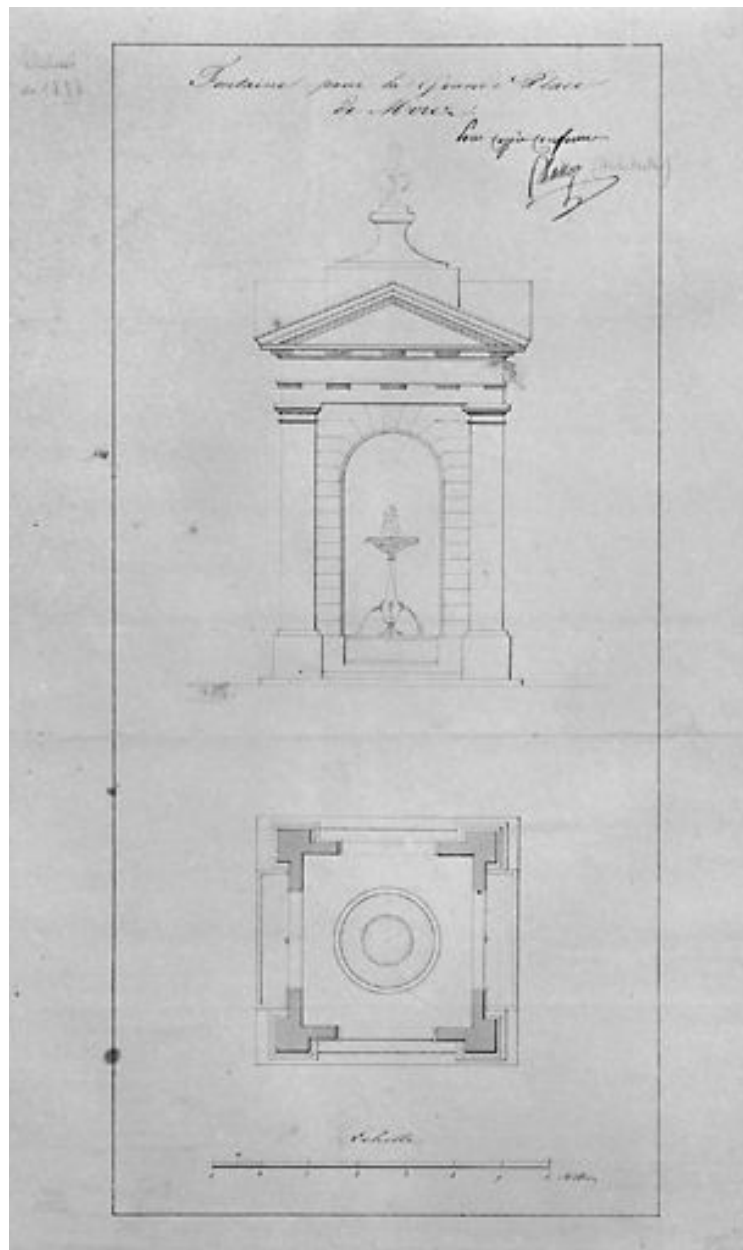
Fontaine pour la Grande Place de Morez [plan et élévation] : dessin (plume, lavis), s.d. [vers 1836], échelle approximative 1:70.
