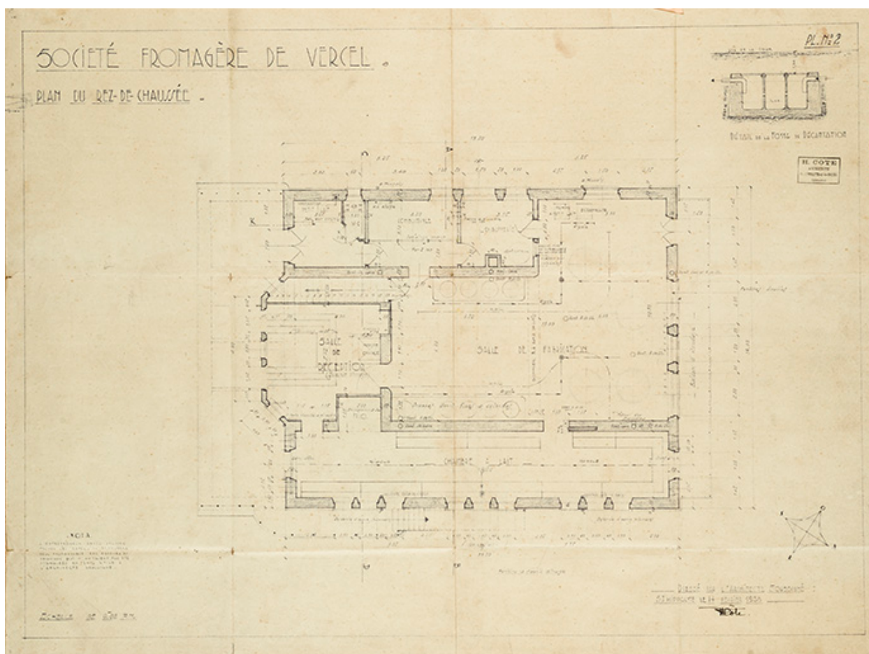
Soci t  fromag re de Vercel. Plan du rez-de-chauss e, 1938.
