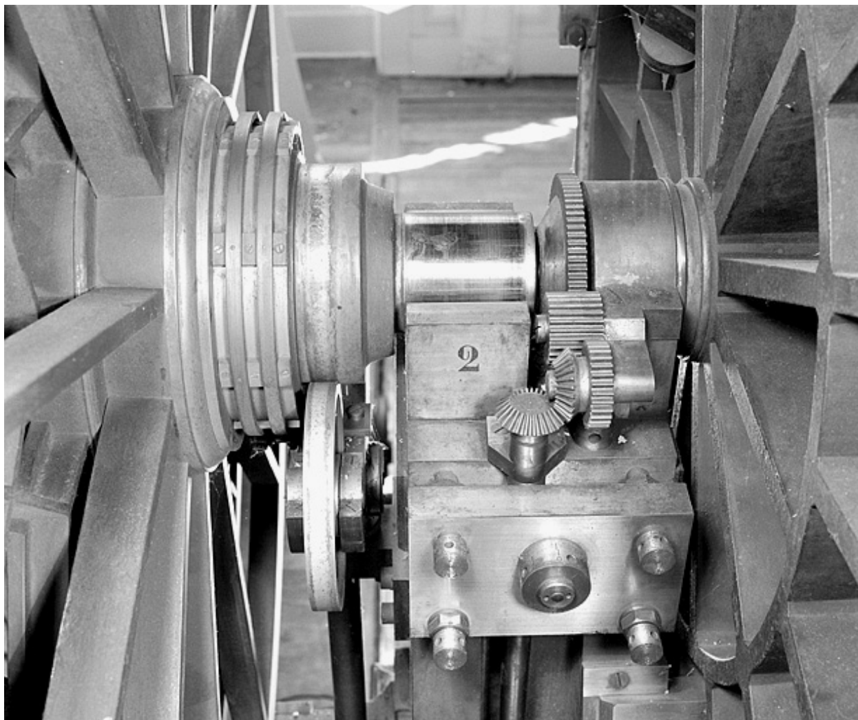
Axe des tourillons.
