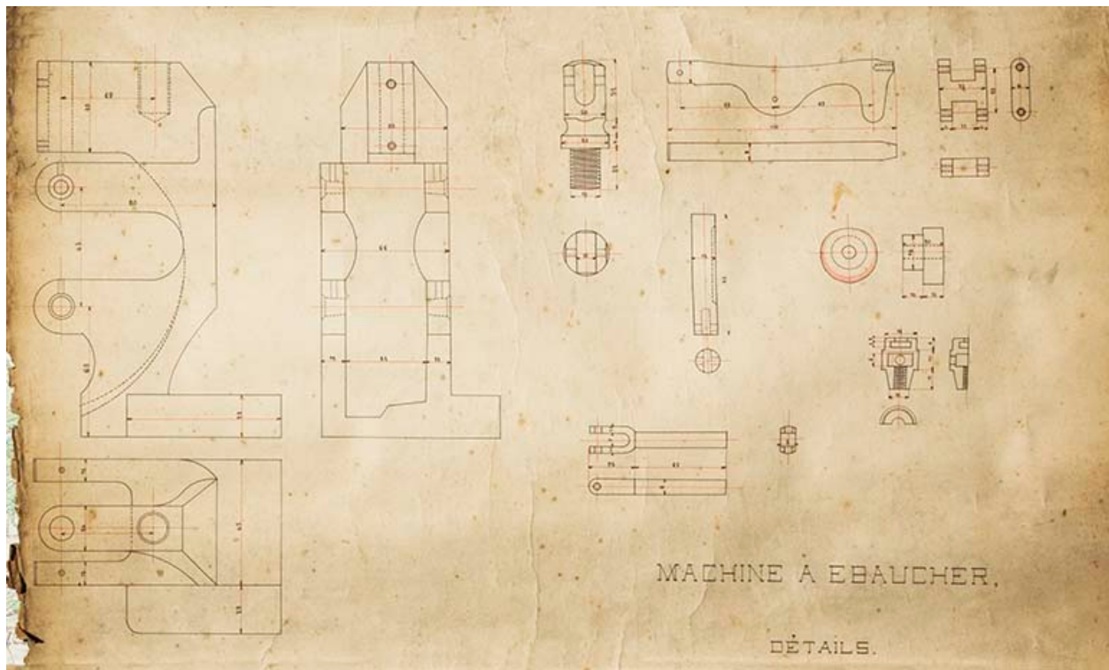
Machine à ébaucher. Détails, 1916.
