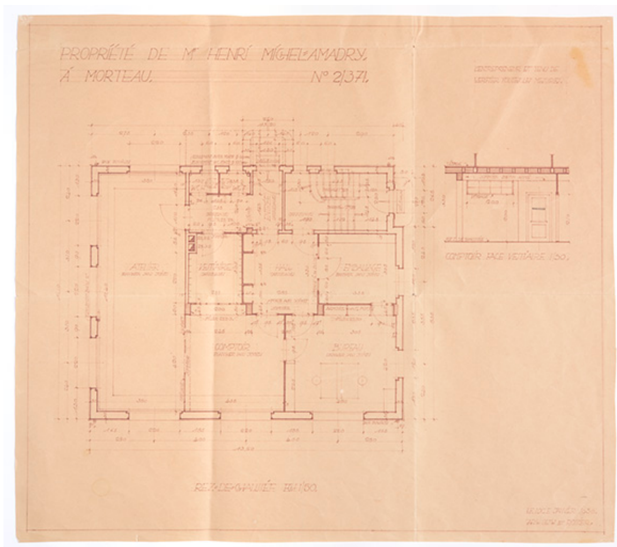
Propriété de Mr Henri Michel-Amadry, à Morteau. Rez-de-chaussée [plan et] Comptoir face vestiaire [élévation], janvier 1930
