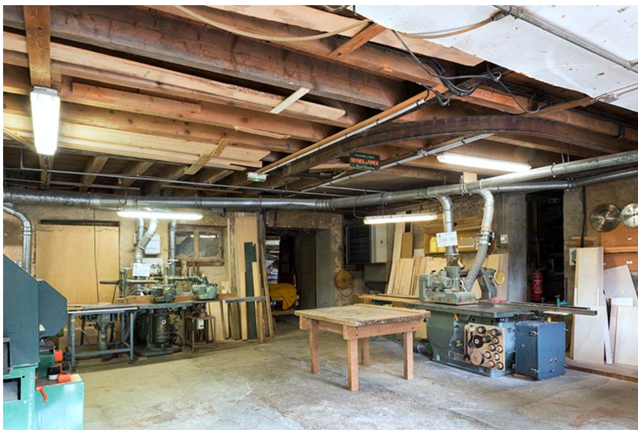
Atelier de fabrication : vue intérieure au rez-de-chaussée.
