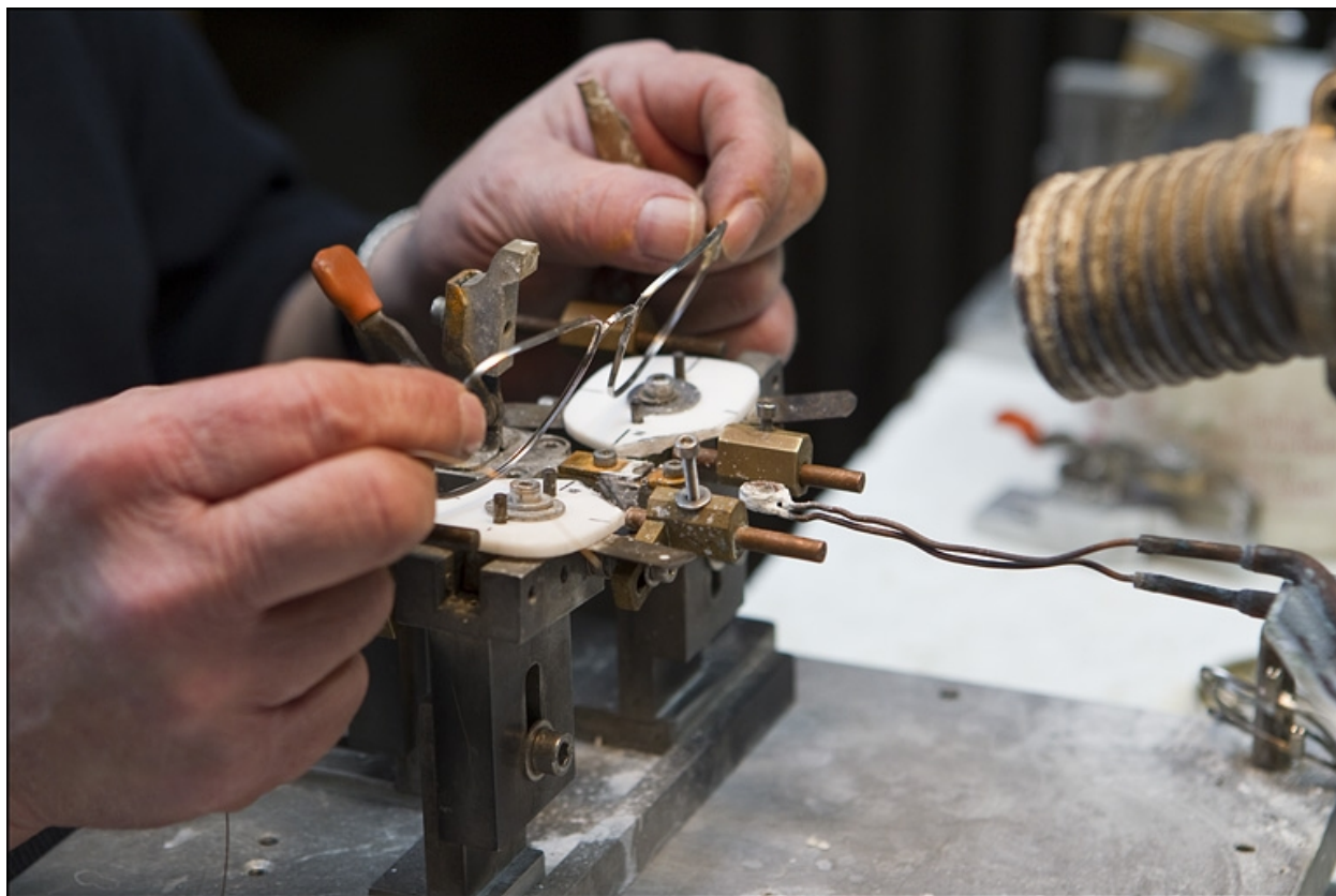
Usine Gouverneur-Audigier, Morez : soudage sur la machine à souder Himmel.
