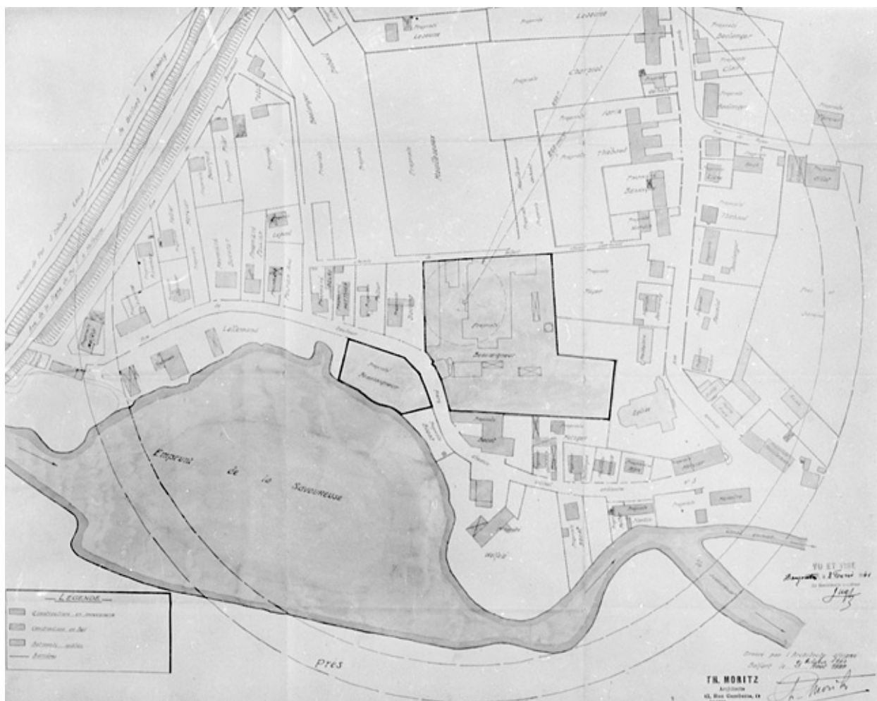
Etablissement J. Beauseigneur à Danjoutin (Territoire de Belfort) Ancienne Teinturerie Alsacienne - Plan d'ensemble de la propriété.
