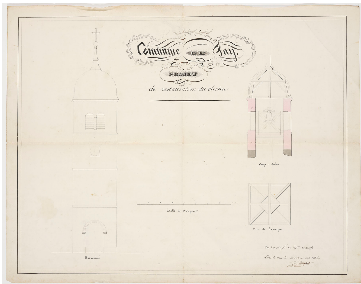
Projet de restauration du clocher. Elévation. Coupe du clocher. Plan de l'enrayure. 1838.
