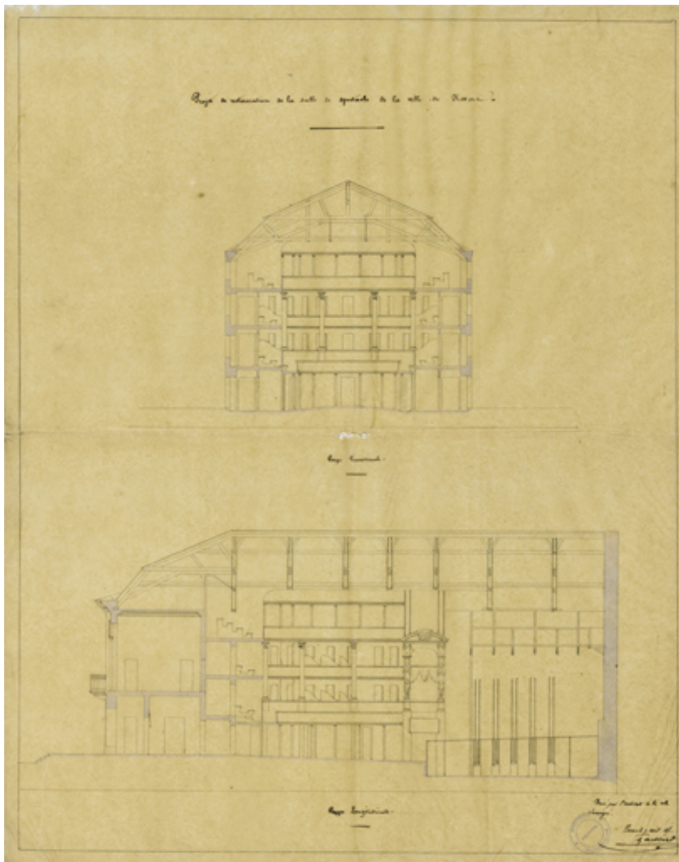
Projet de restauration de la salle de spectacle de la ville de Nevers. Coupe transversale [et] Coupe longitudinale. 9 avril 1851.
