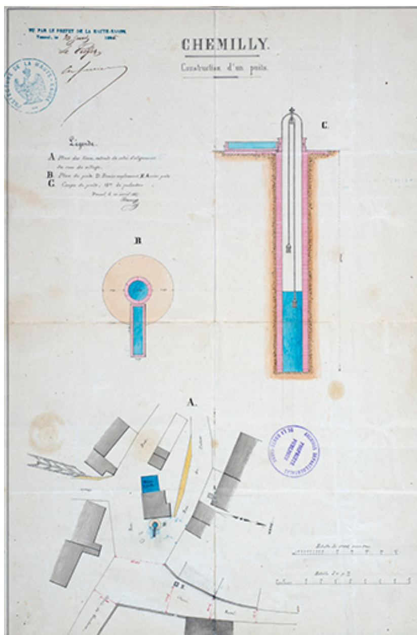
Plan de situation et plan en coupe du puits à reconstruire, 1865
