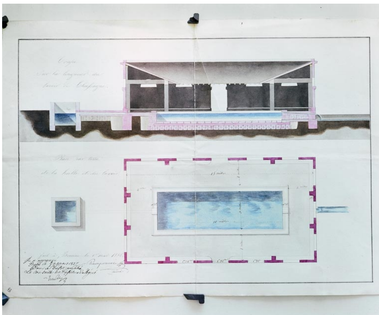
Plan et coupe longitudinale, devis daté du 1er mai 1836 par Champonnois aîné (architecte).
