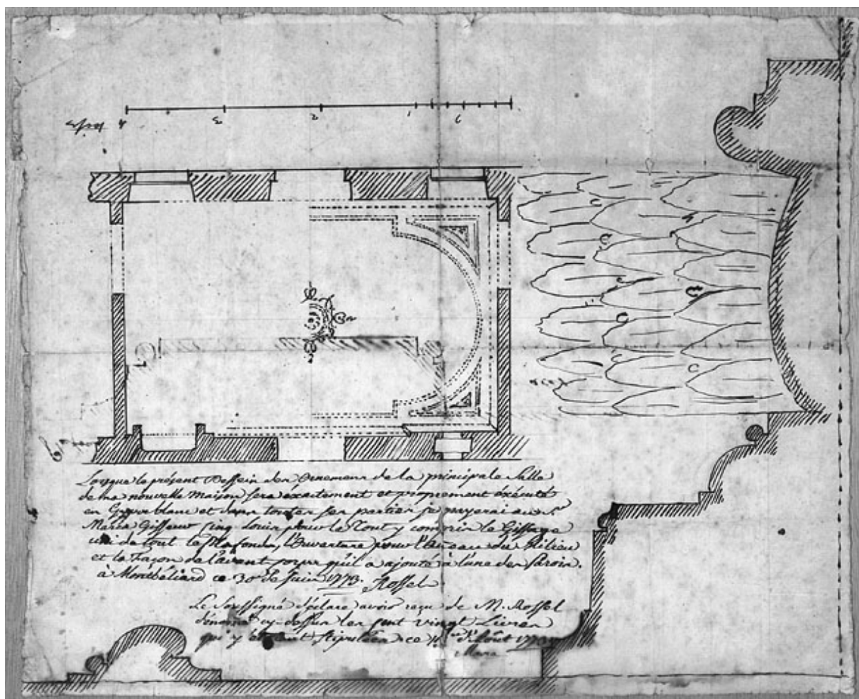
Plan du décor du plafond du grand salon, coupes des moulures, détail de la frise, 1773.
