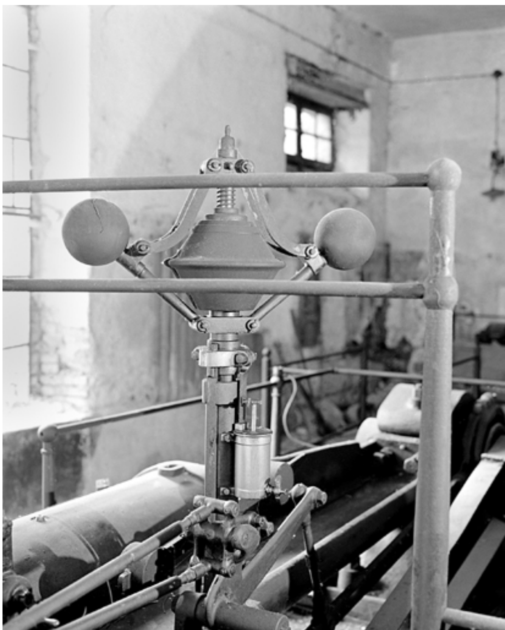
Régulateur à boules.
