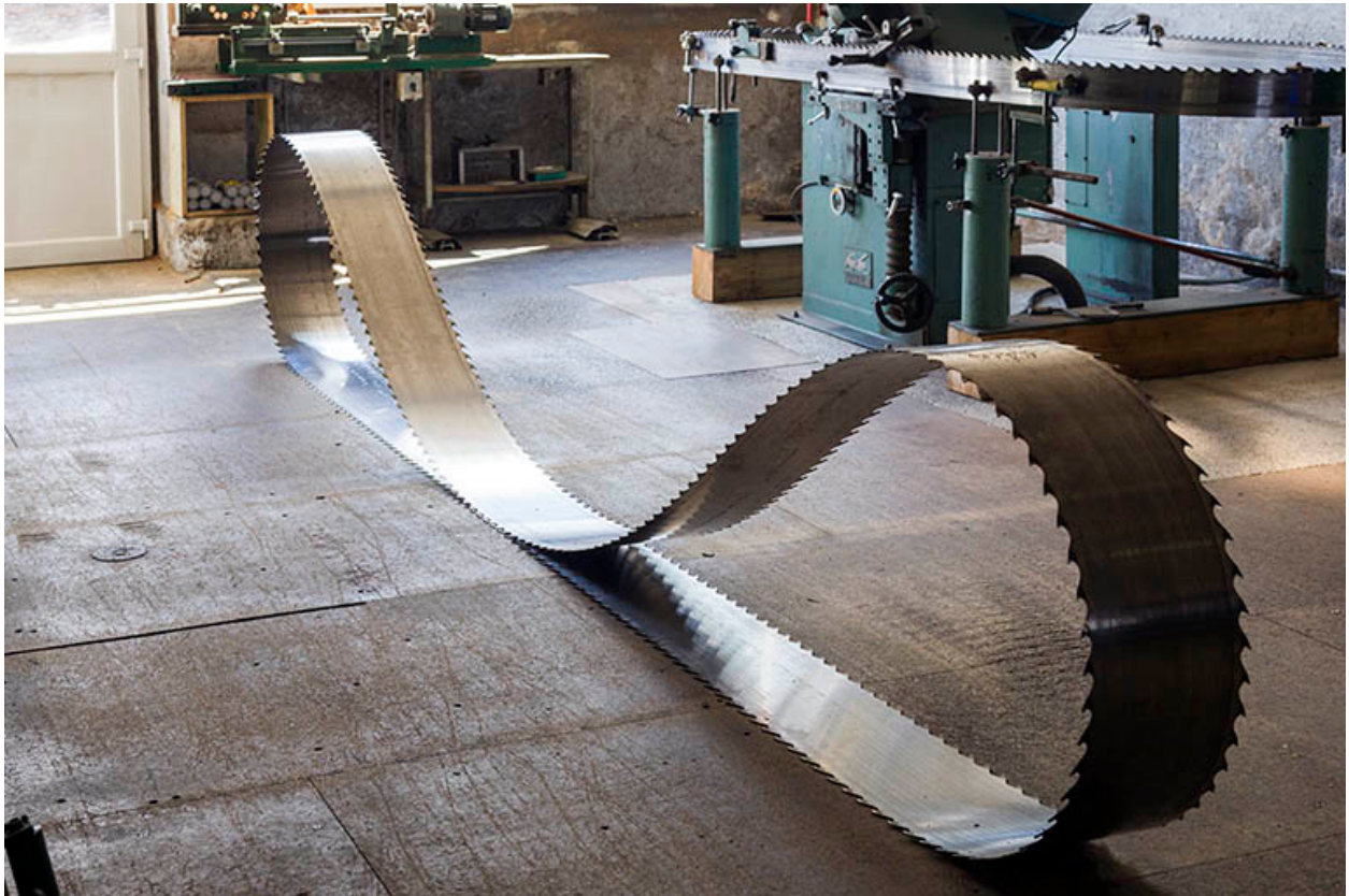
Atelier d'affûtage (K) : lame de scie à ruban à double denture.
