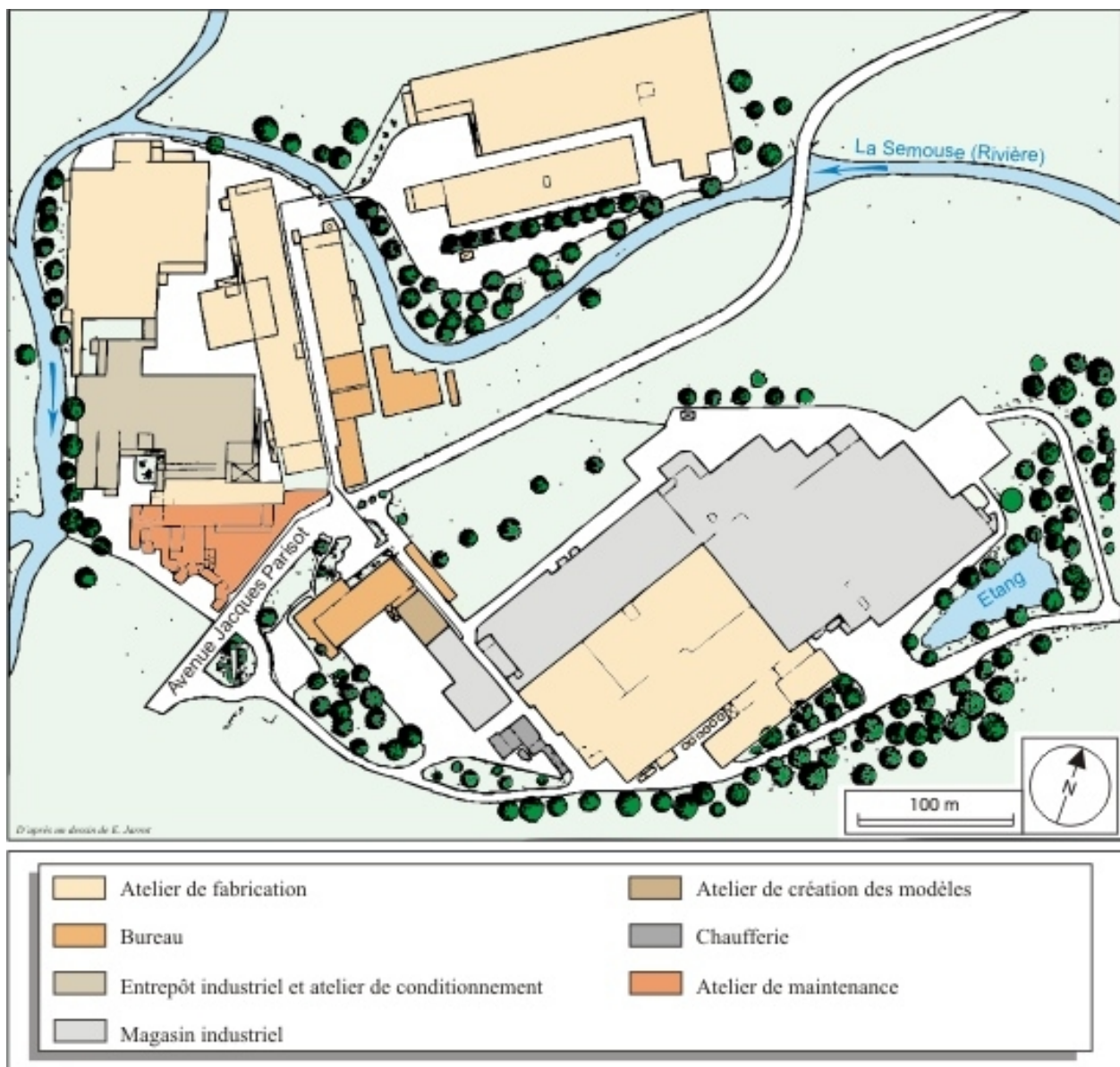
Plan-masse de l'usine. D'après un plan de l'entreprise, mis au net par André Céréza.
