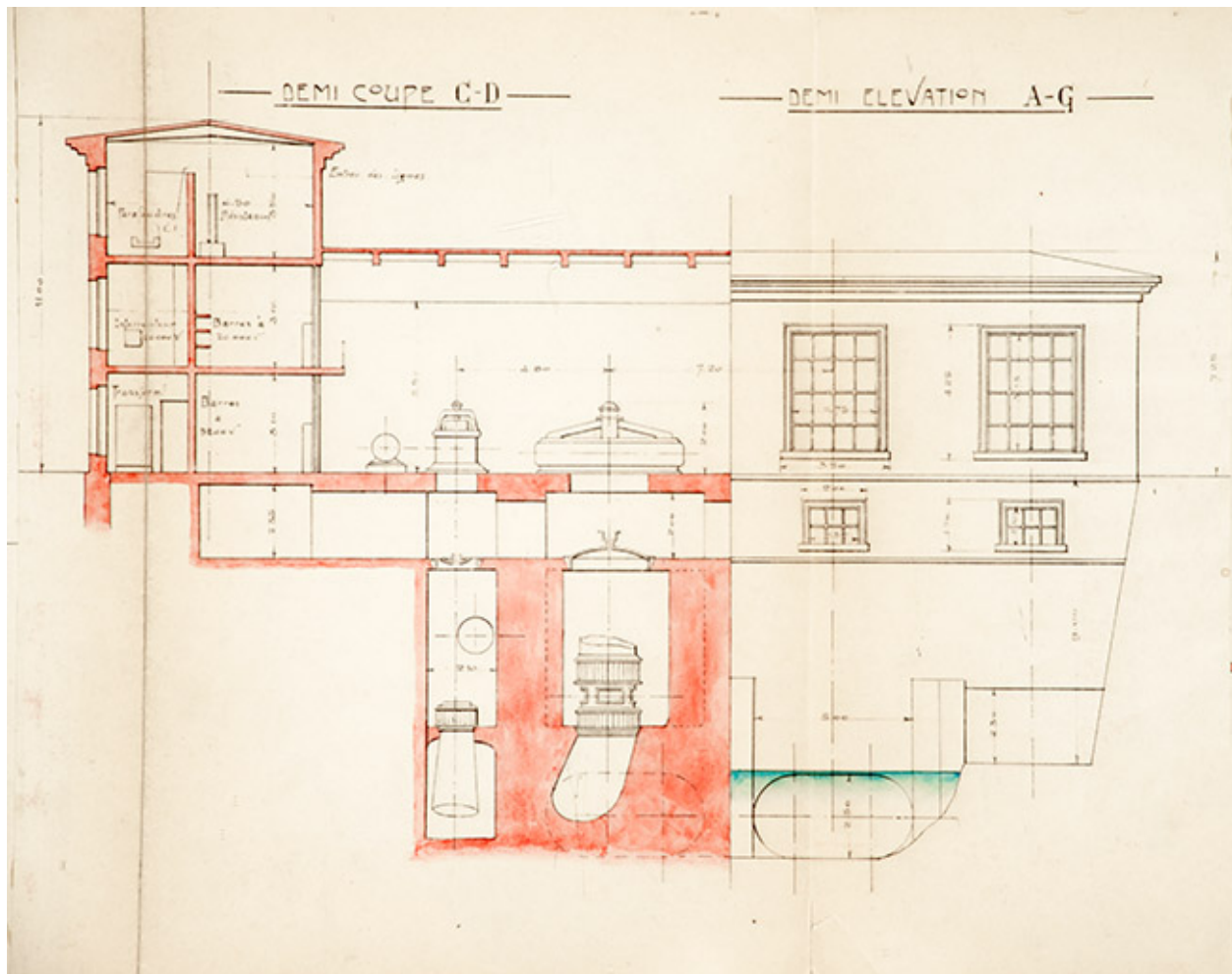
Usine électrique du Châtelot, demi-coupe et demi-élévation, 1917.
