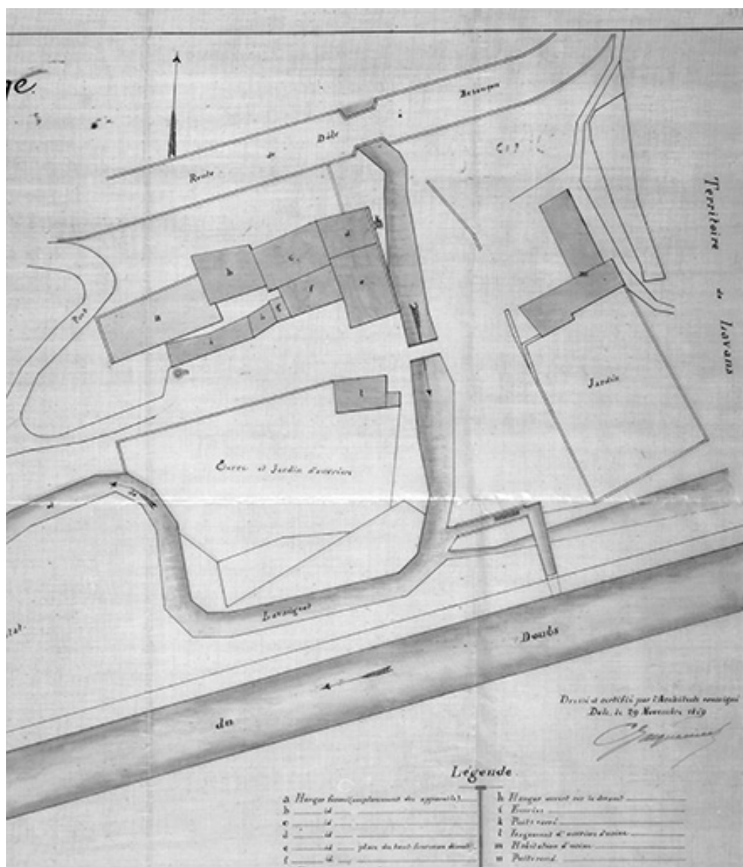
Usine du Moulin-Rouge. Plan général.
