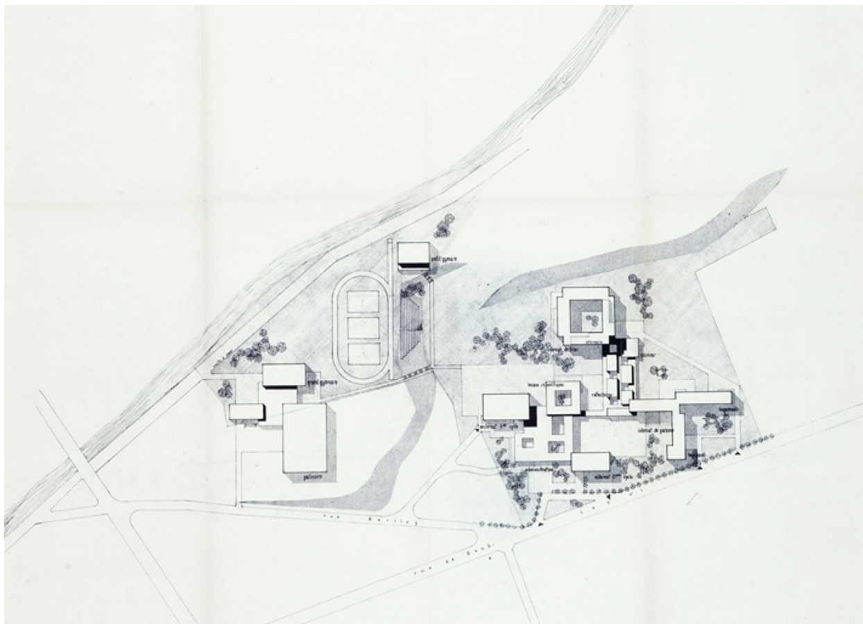
Lycée mixte de Pontarlier. Esquisse n° 3 EP 04. Plan-masse. Juillet 1964.
