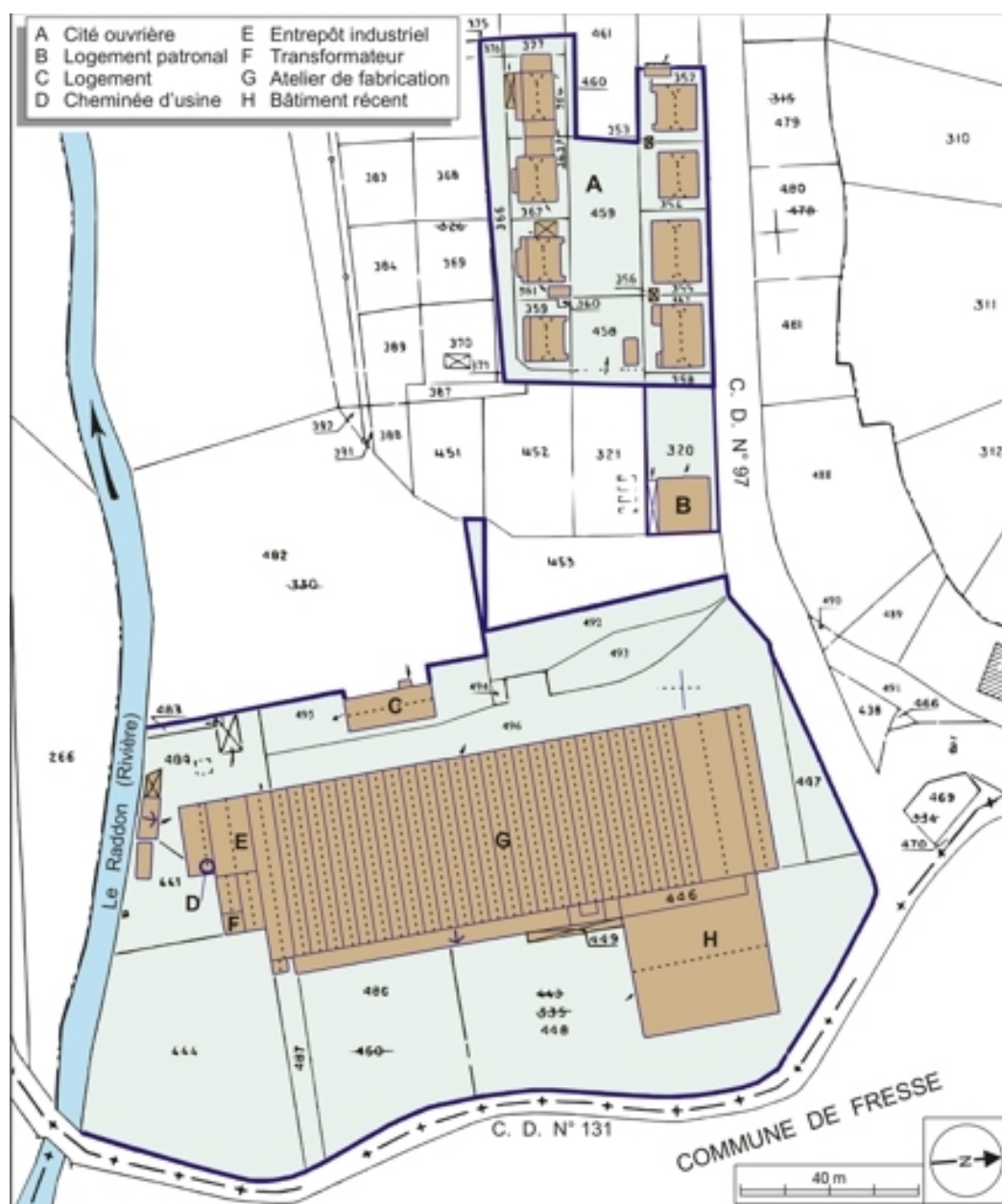
Plan-masse et de situation. Extrait du plan cadastral numérisé, 2005, section B, 1:1000 réduit à 1:1250.
