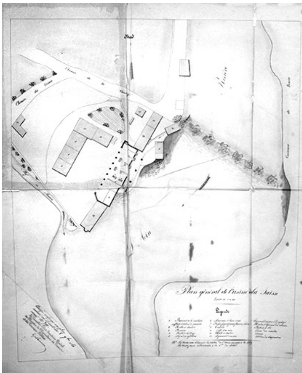
Usine de la Saisse. Plan général [...].
