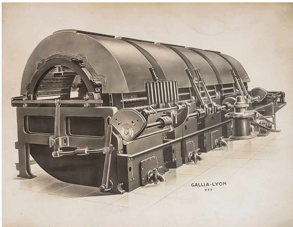
Modèle de machine de trempage (Gallia-Lyon 777).
