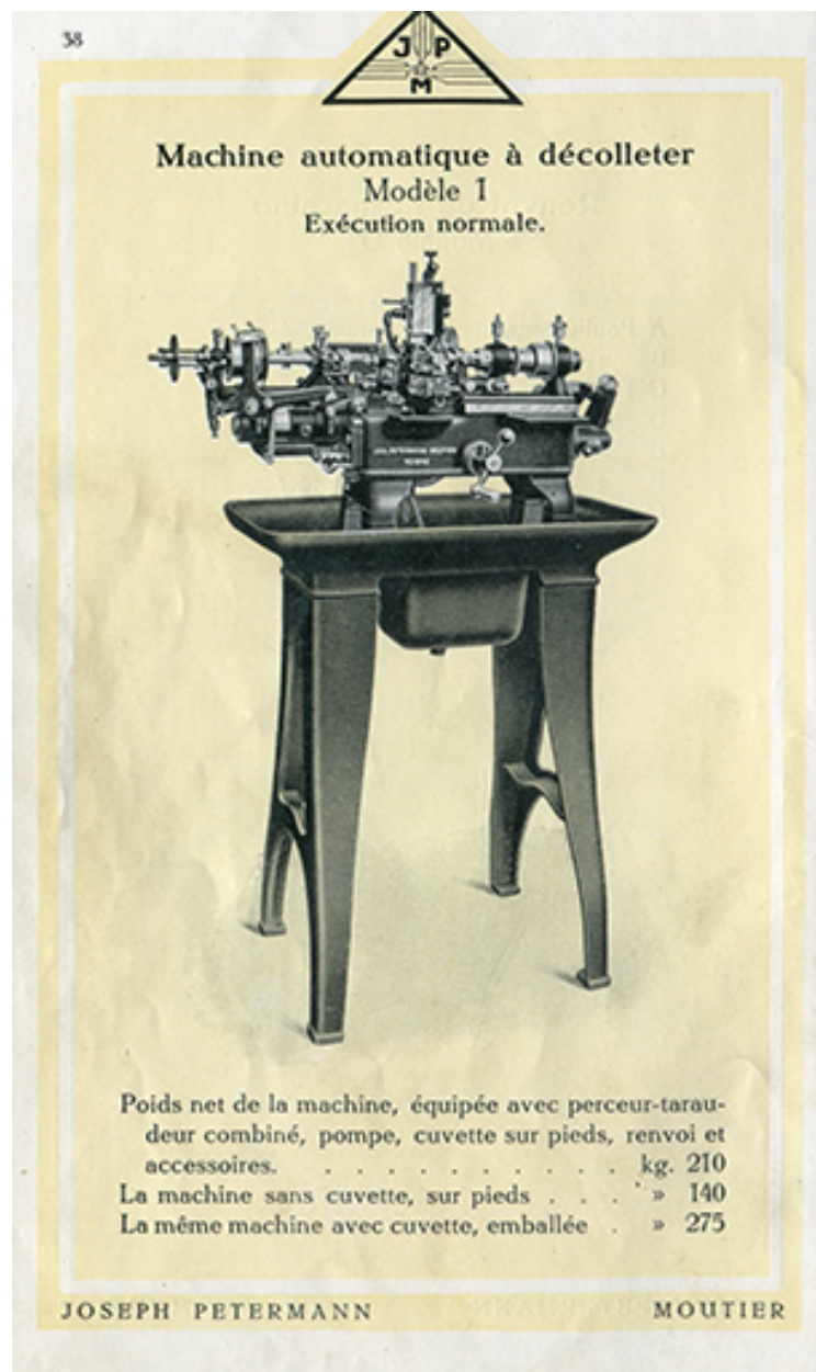
Machine automatique à décolleter modèle 1, exécution normale, années 1920.
