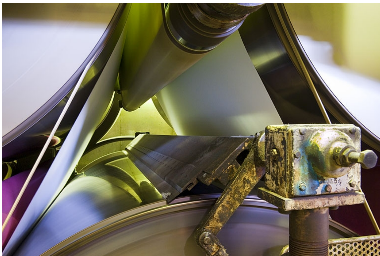
Papeterie de Mandeure. Séchage de la feuille dans la machine à papier.
