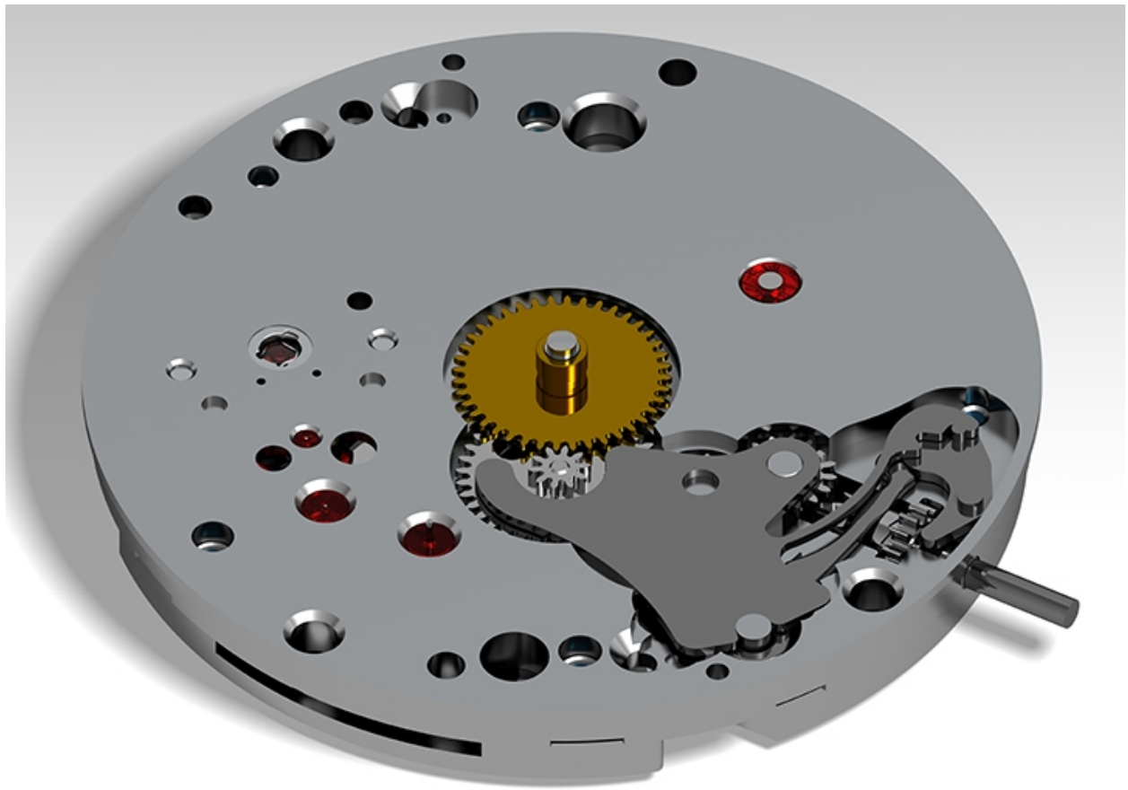
Montre de gousset mécanique : mouvement côté cadran.
