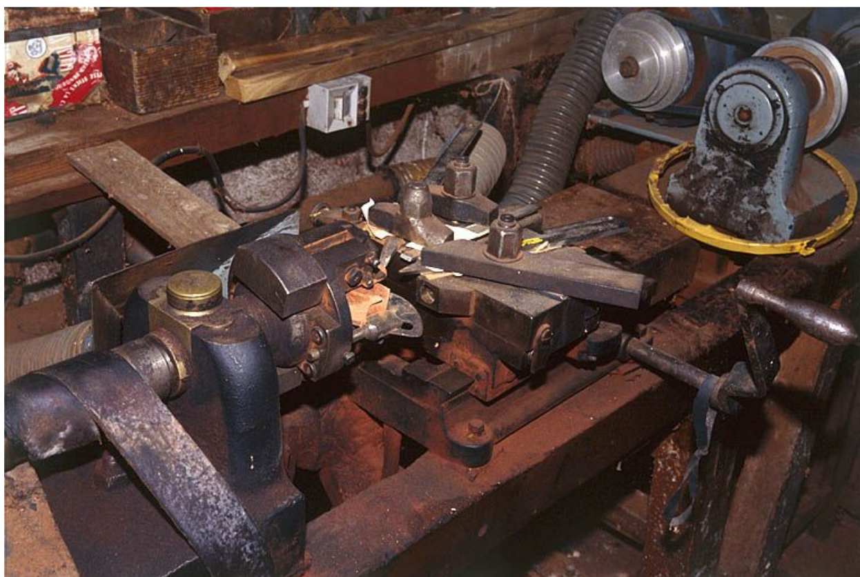
Mandrin gueule de loup et chariot porte-outils.
